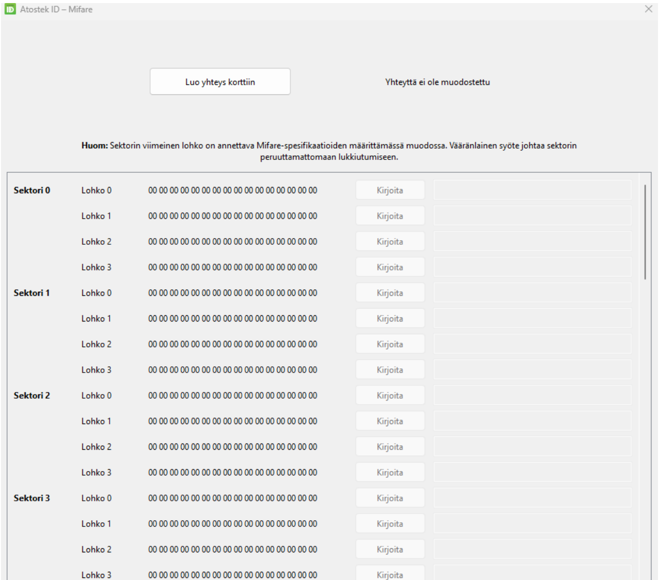
Kuva 15. Mifare-sirun hallintanäkymä.
